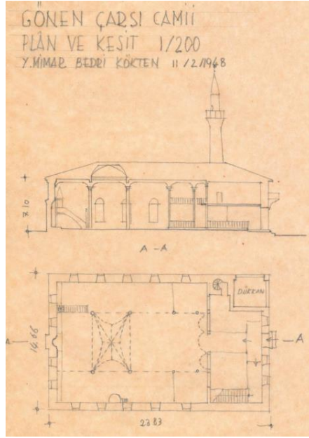
1948 Yılına Ait Gönen Çarşı Camisine Ait Çizim
